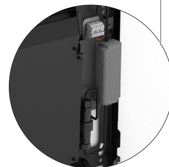
AANSLUITING 230 VAC MET WATERDICHTE VOEDING EN AANSLUITWARTEL
